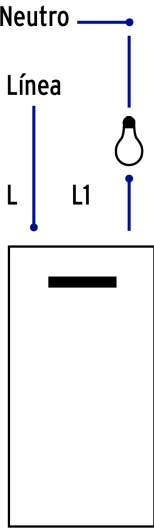
Diagrama de conexión
