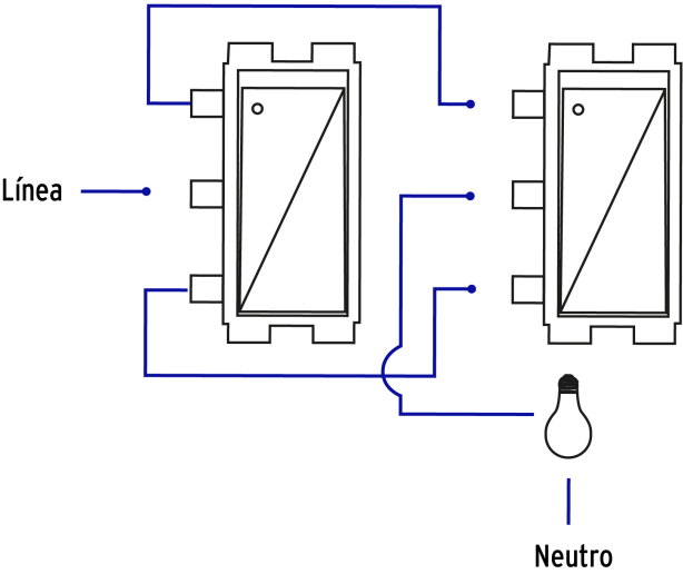
Diagrama de conexión
