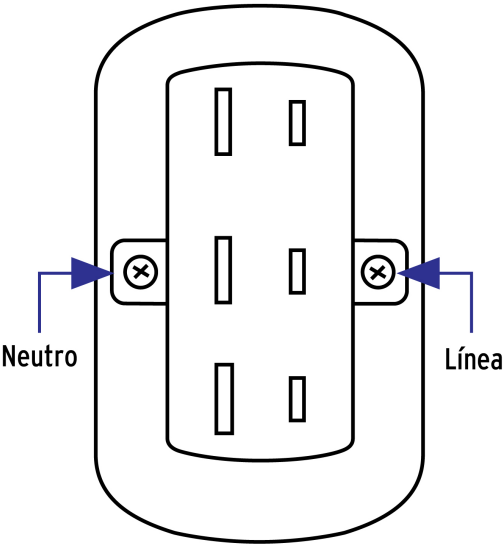
Diagrama de conexión
